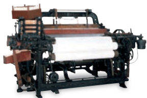
無停止杆換式豊田自動織機 (G型)
