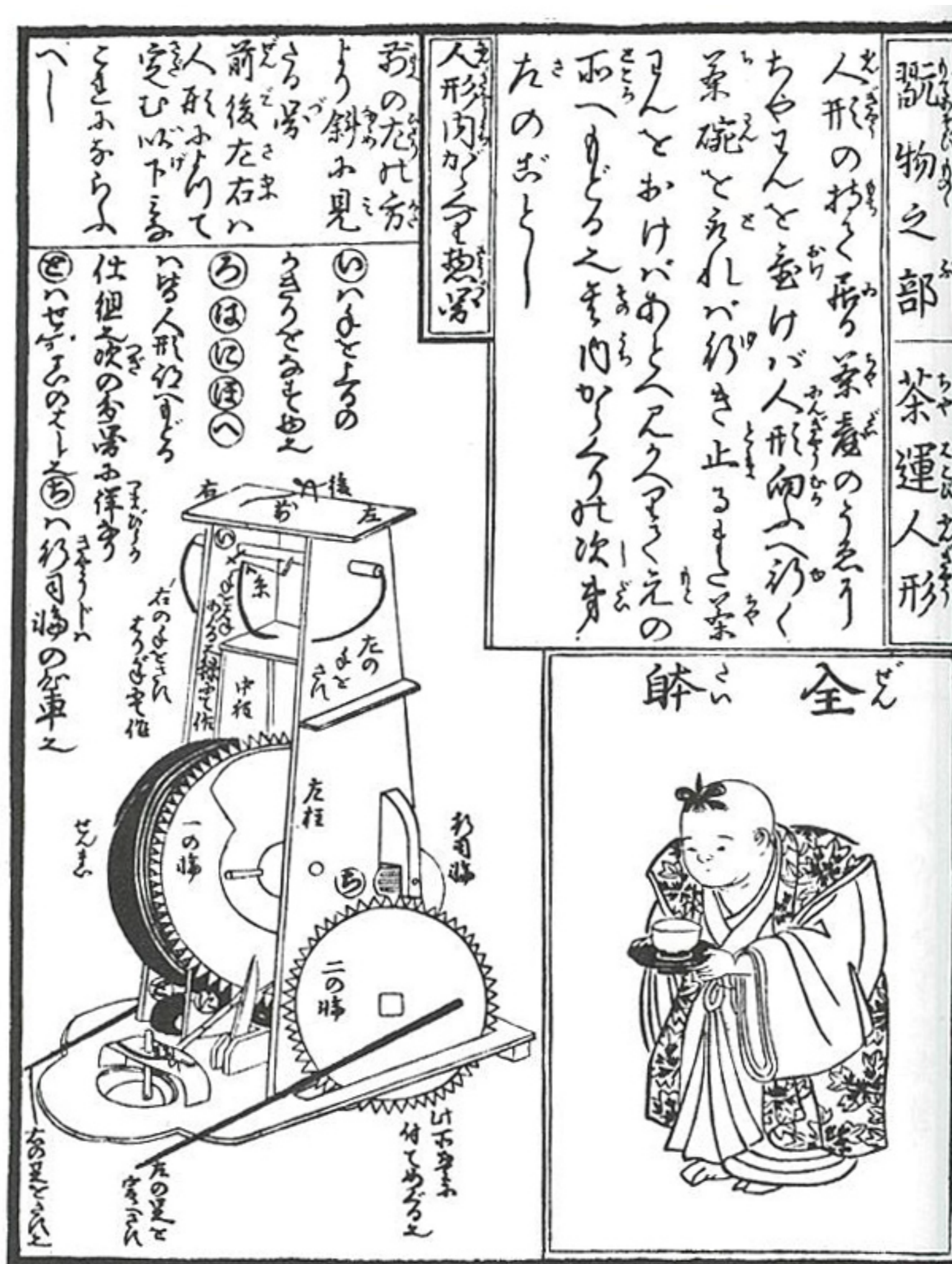
からくりずい 細川半蔵『機巧図彙』
